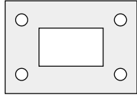
Fodplade 200 x 300 x 20 mm (Måling nr. 1, 2)
